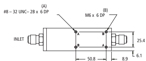
M100M Ansicht von unten
