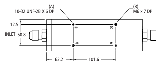
C100H1, H2 Ansicht von unten
