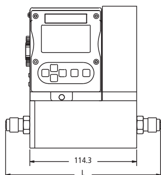
C100M Vorderansicht
