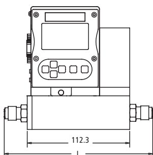
C100 High Pressure Vorderansicht
