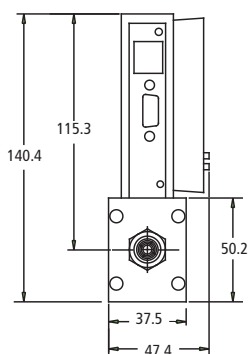
M100M Einlass Ansicht
