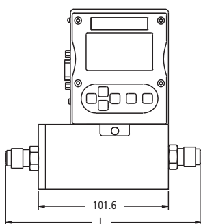
M100M Vorderansicht
