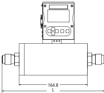
M100H Vorderansicht
